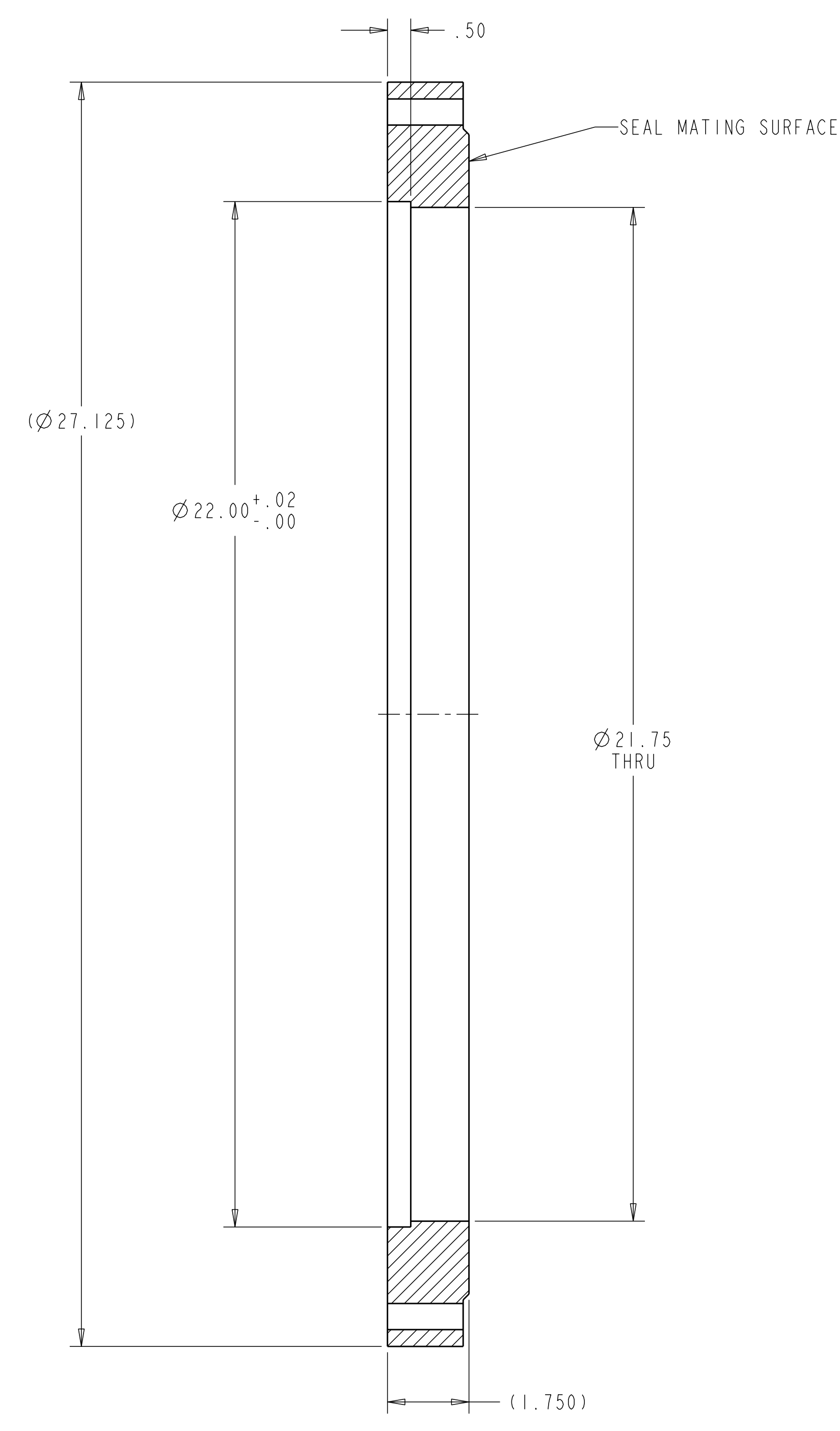
SECTION A-A
