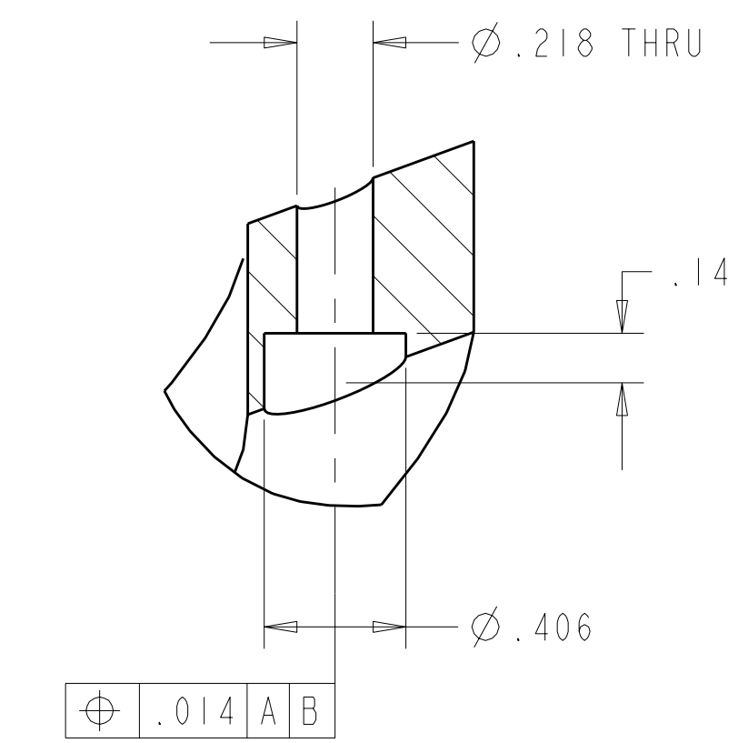
SECTION A-A TYP 8X SCALE 2.000
