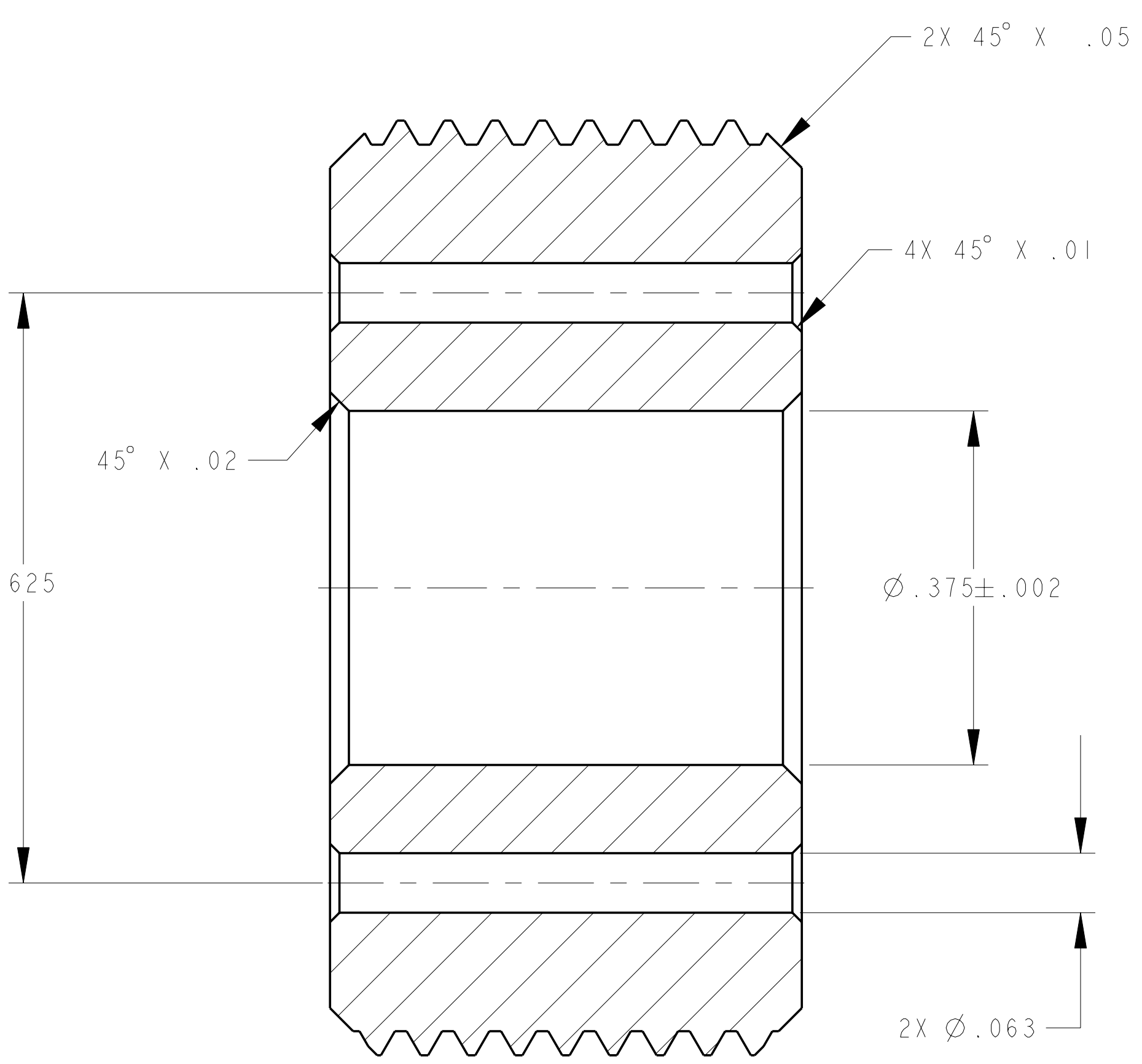
SECTION A-A
