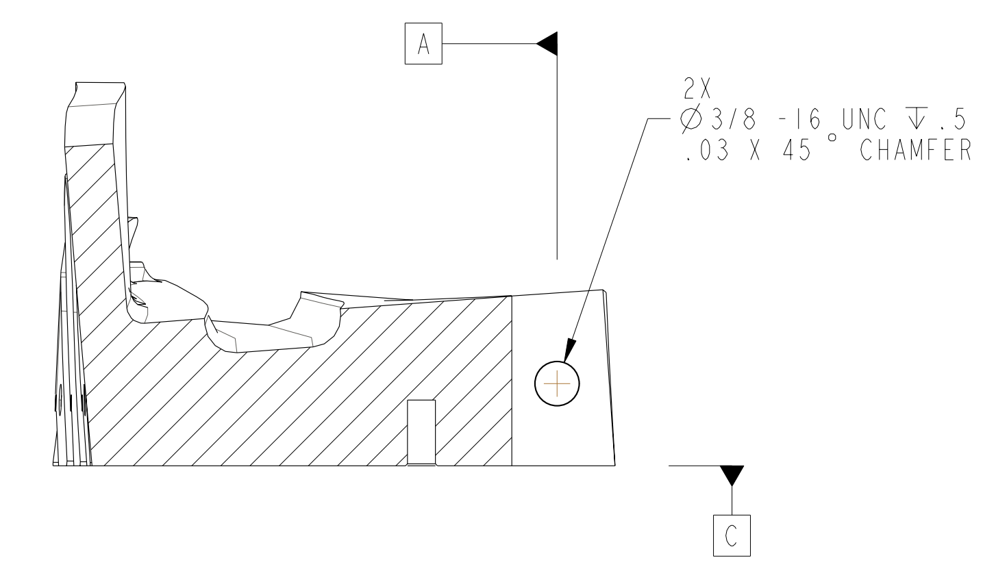
SECTION A-A
