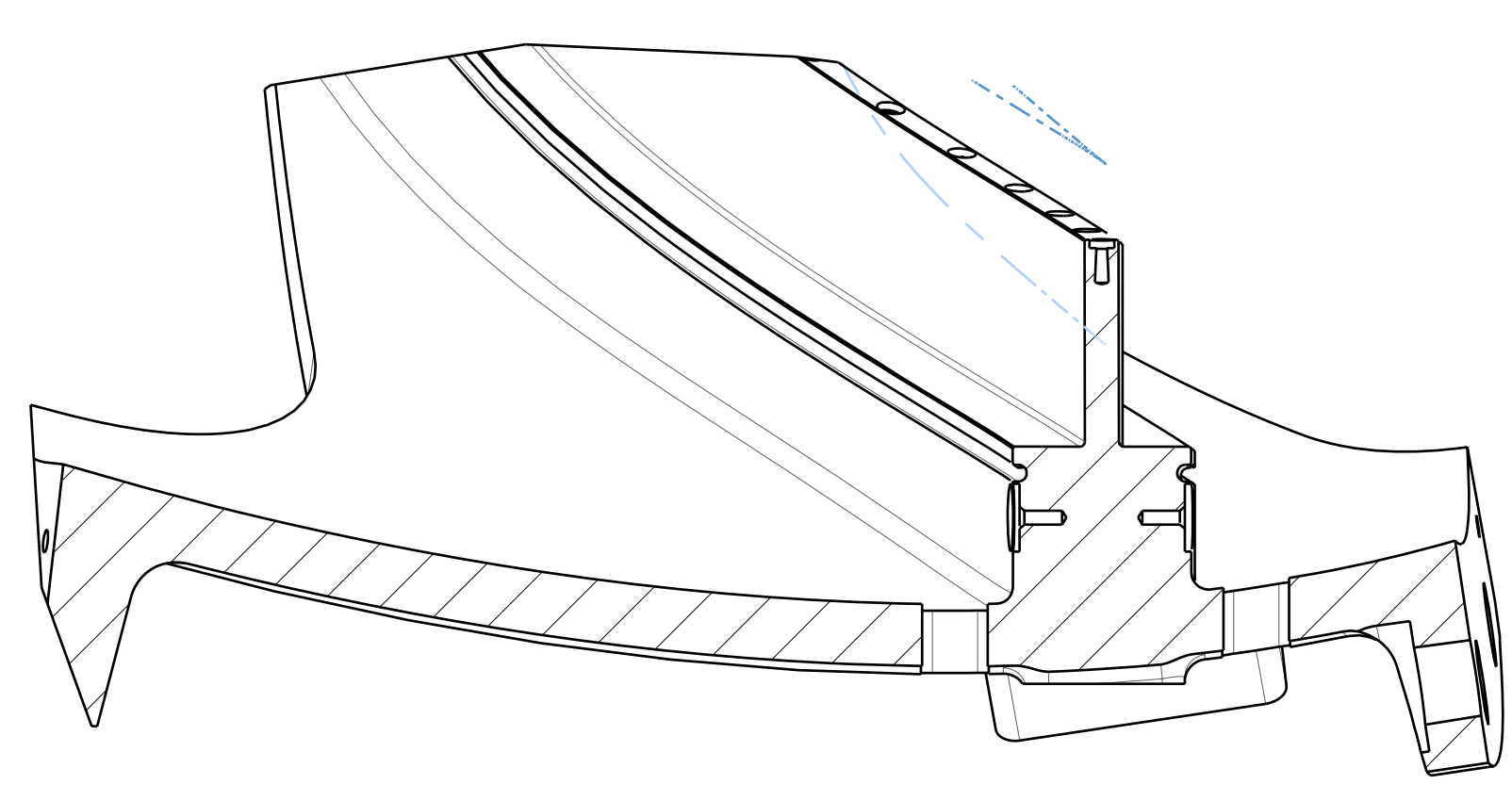
SECTION G3-G3
