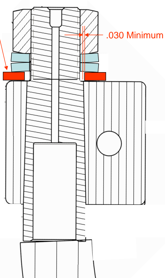
Lug Assembly
