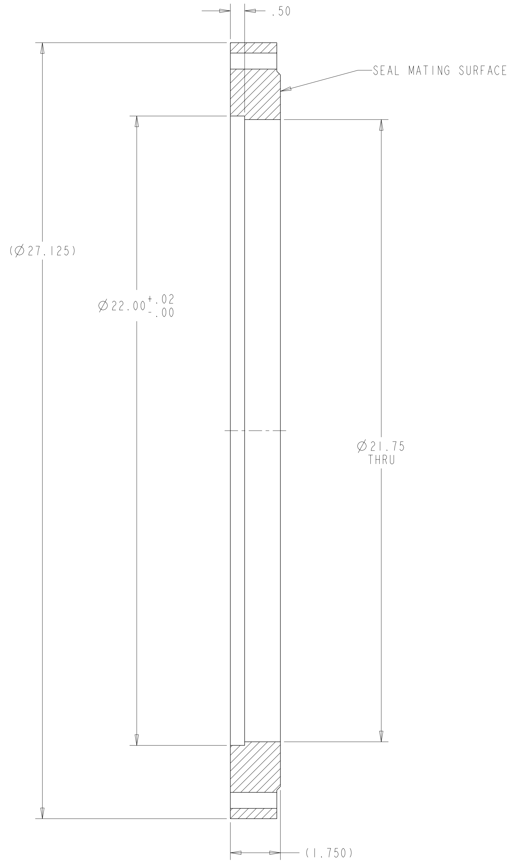
SECTION A-A
