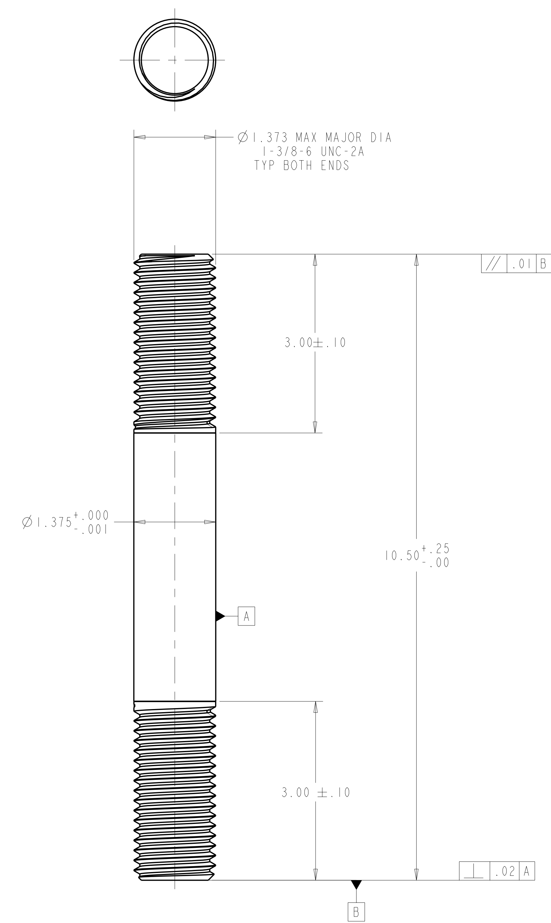
-1 MCWF FLANGE STUD SCALE 1.00
