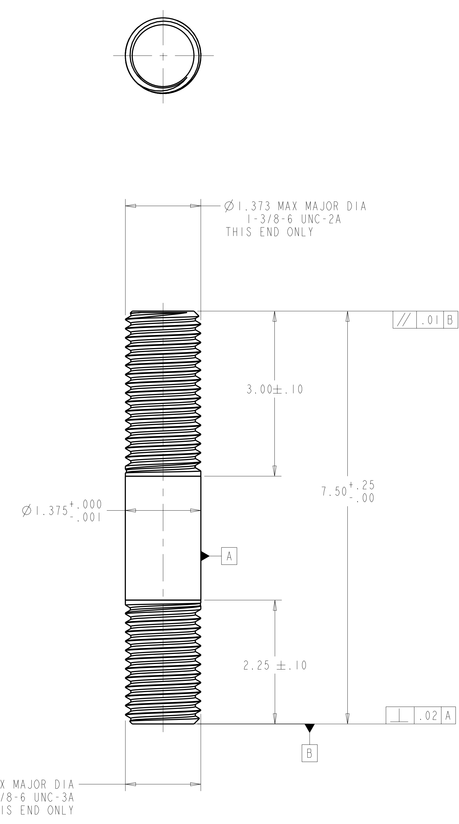
-2 MCWF FLANGE STUD SCALE 1.00
