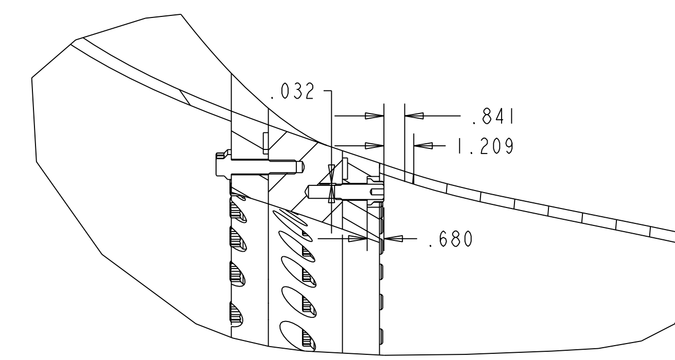
SECTION 15-15
