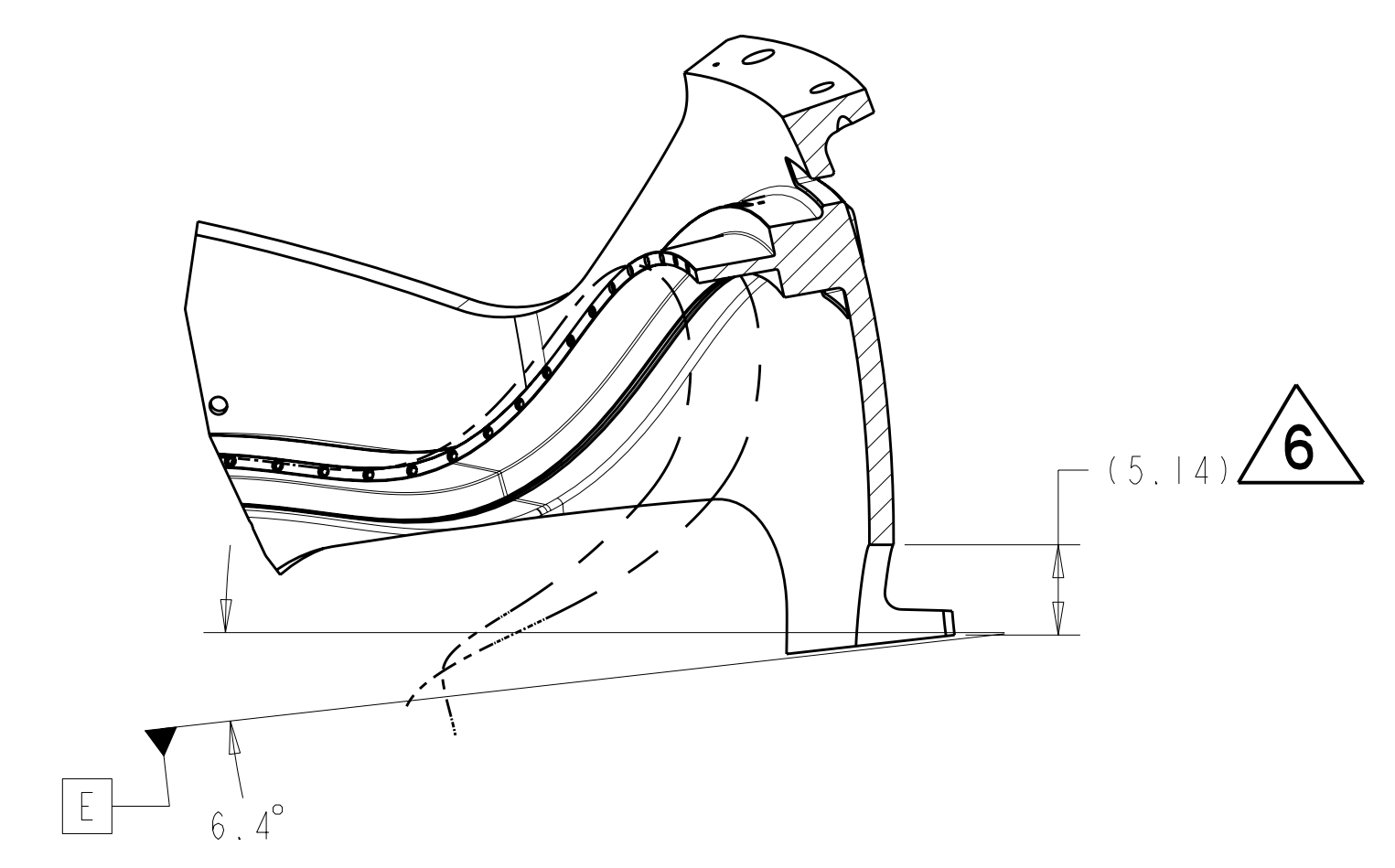
SECTION P5-P5 SCALE 0.1
