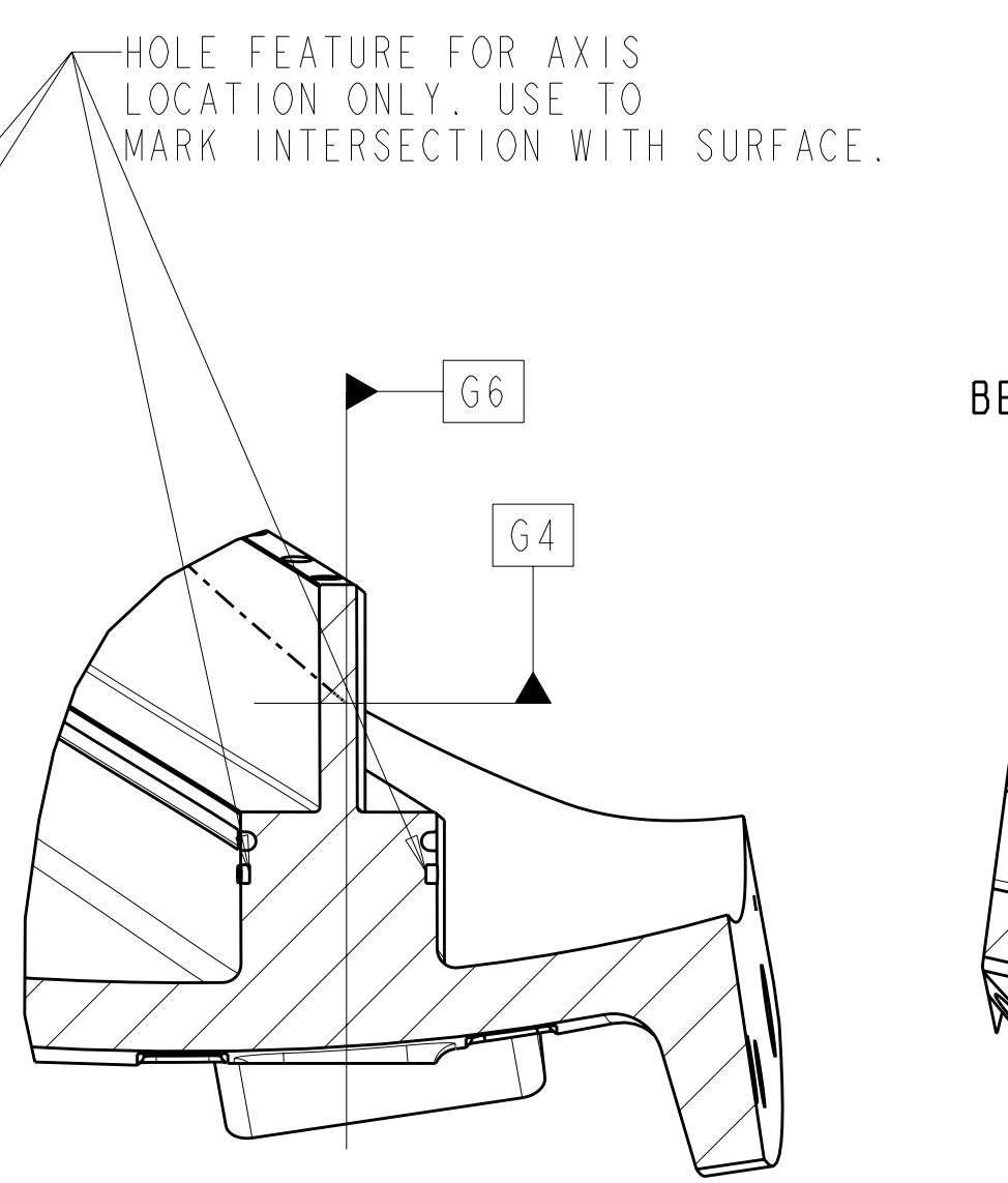
SECTION G3-G3
