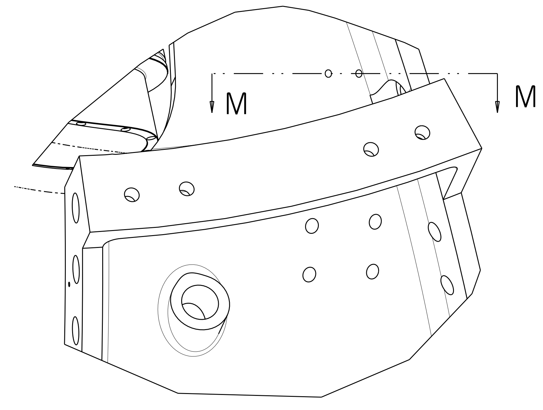
VPI BLEED HOLES
