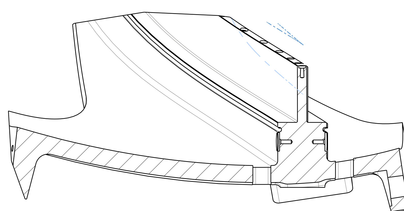
SECTION G3-G3
