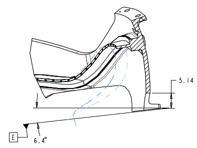
SECTION P5-P5 SCALE 0.1
