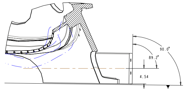
SECTION D1-D1 SCALE 0.19
