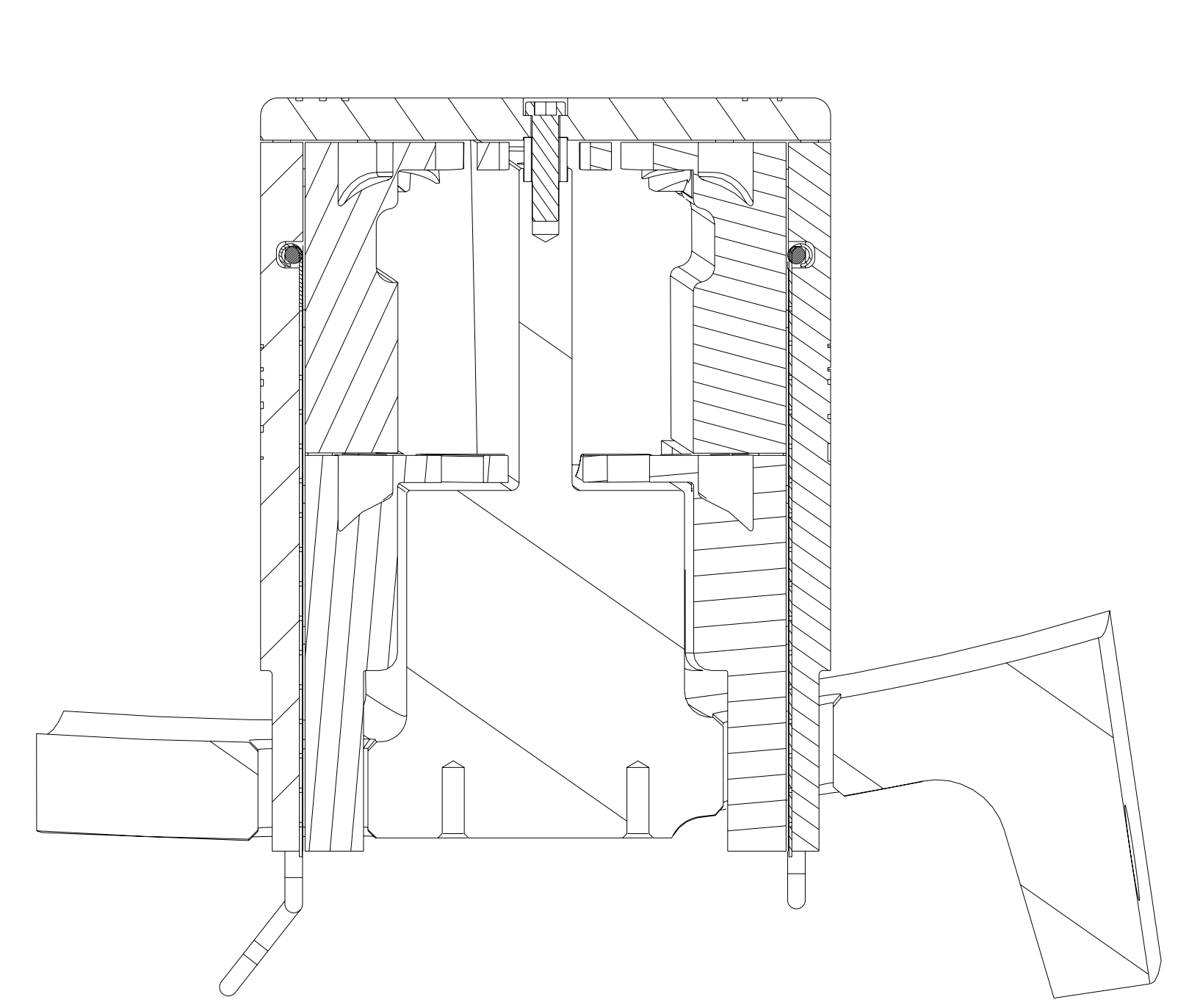
SECTION A-A
