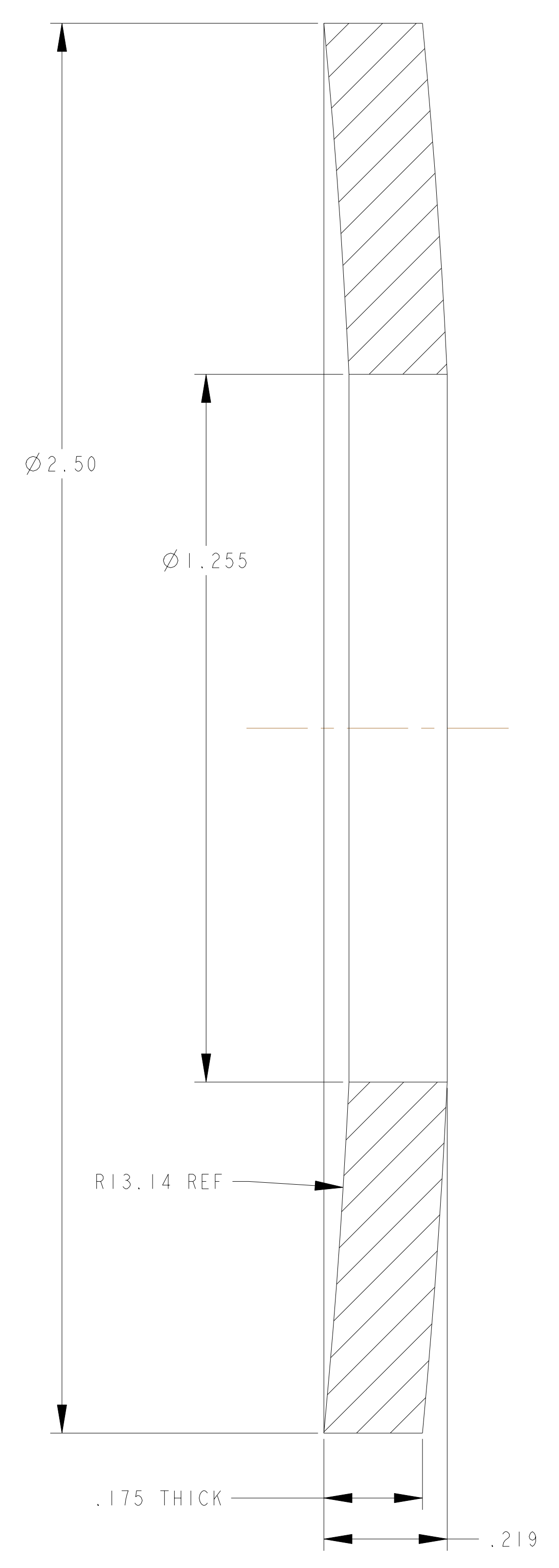
SECTION A-A
