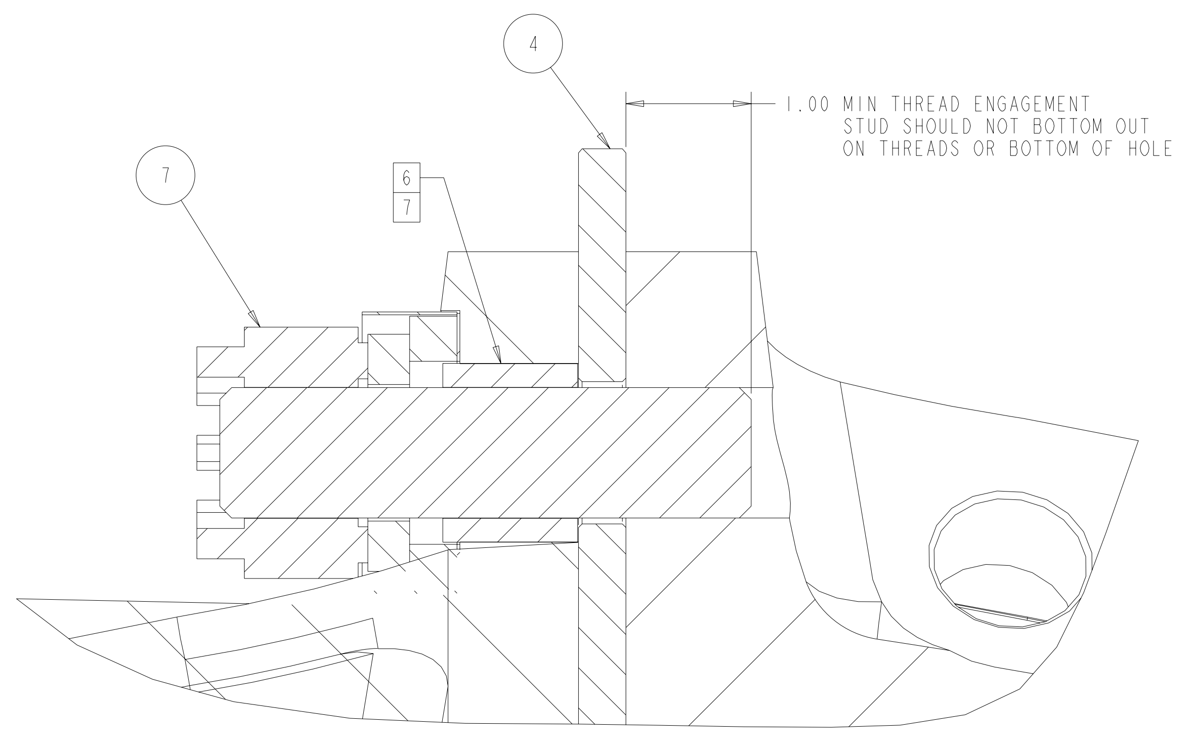
SECTION C-C TYP TAPPED STUD KIT SCALE 1.000
