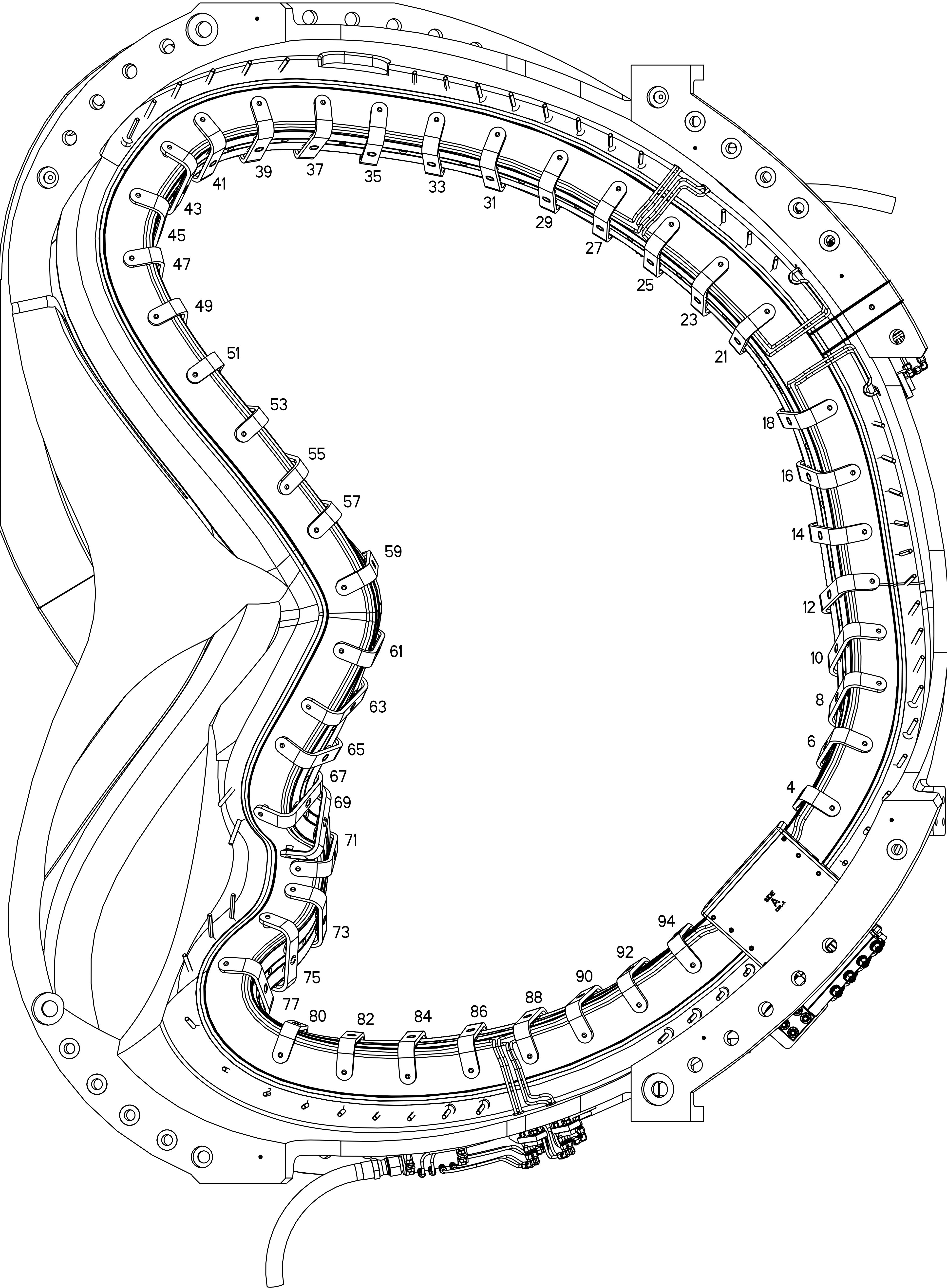
TYPE-A SIDE-A VIEW
