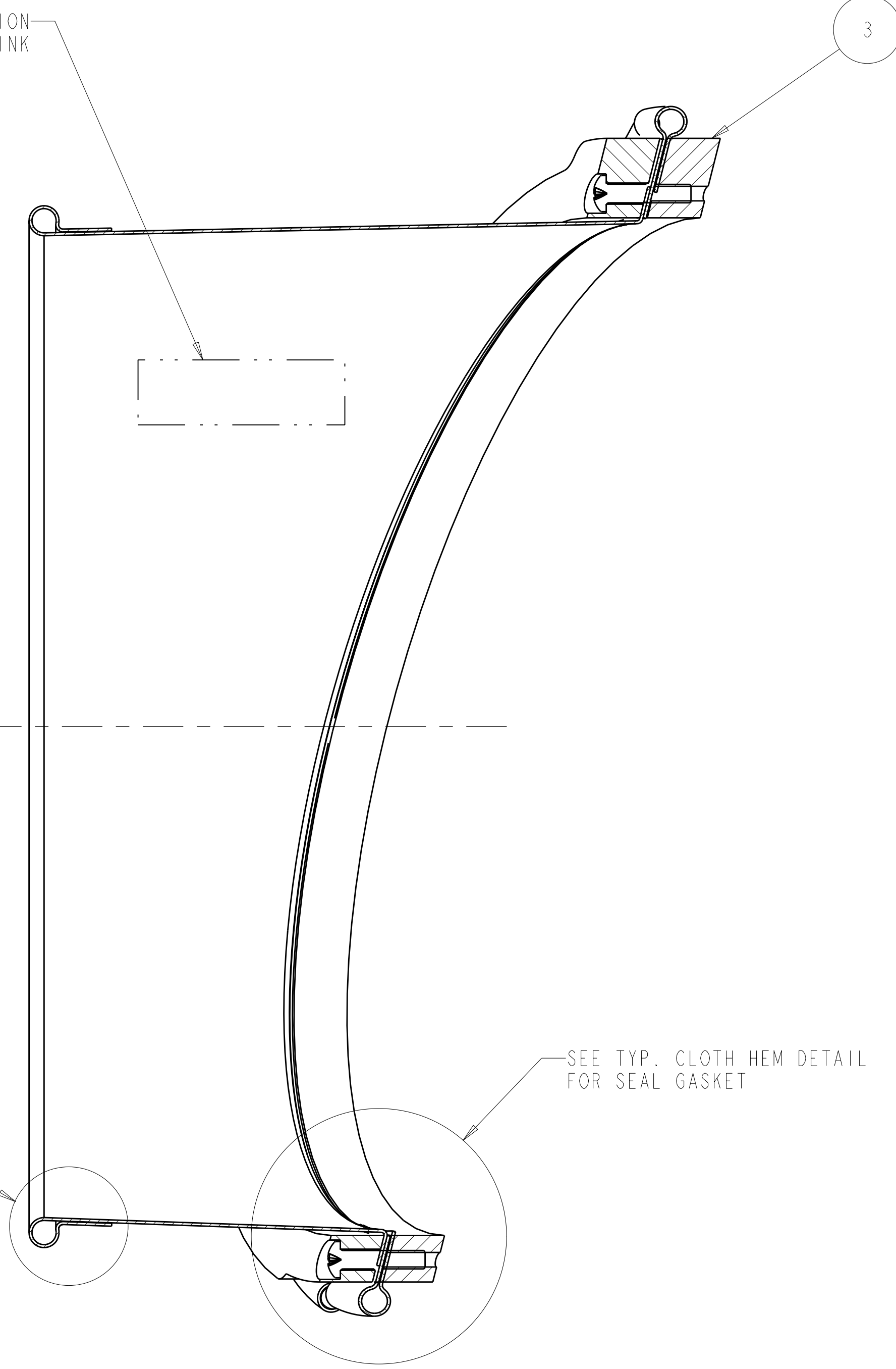
SECTION A-A
