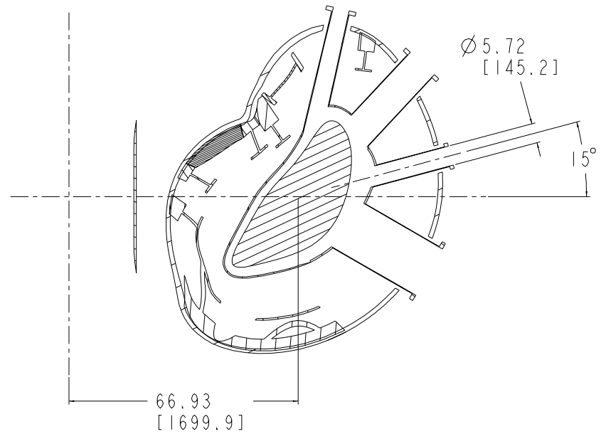
SECTION D-D
