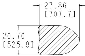
SECTION 60-60
