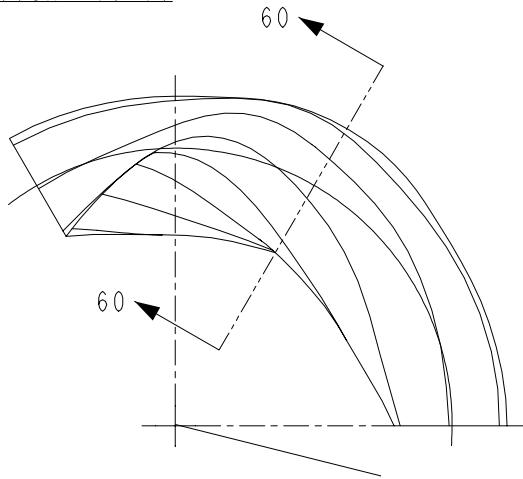
SECTION 60-60
