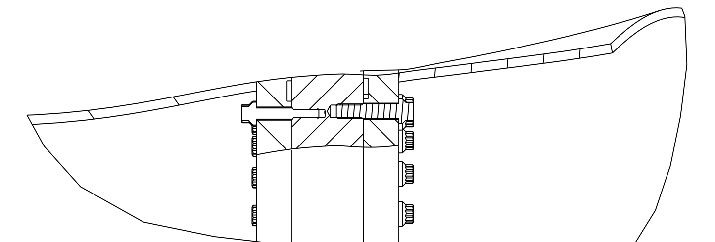
SECTION 25-25
